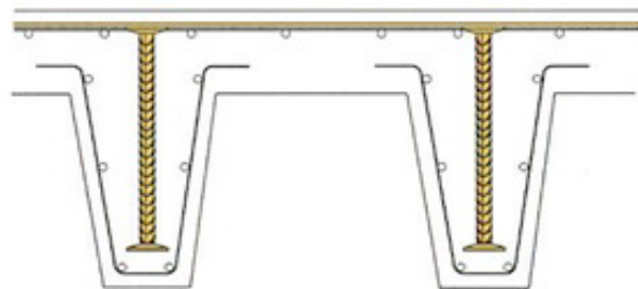
Einbau in Deckenunterzügen (als Schubbewehrung) Installation in beams (as shear reinforcement)
