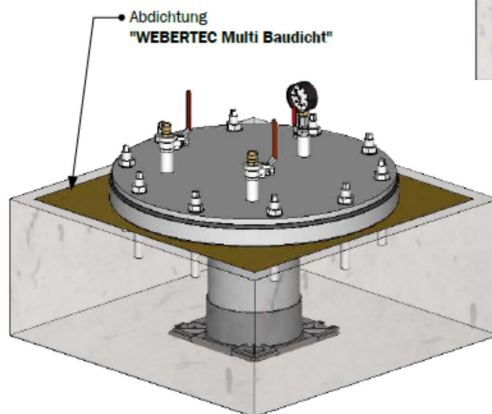
Isometrische Perspektive
