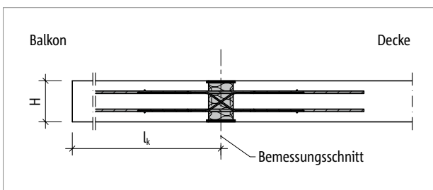
Abb. 314: Schöck Isokorb® XT Typ D: Statisches System
