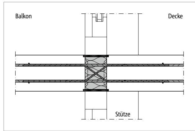
Abb. 312: Schöck Isokorb® XT Typ D: Einbauschnitt; Flachdecke
