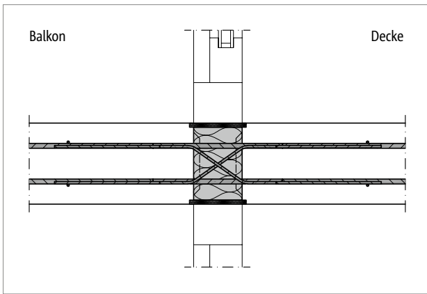
Abb. 311: Schöck Isokorb® XT Typ D: Einbauschnitt; einachsrig gespannte Decke
