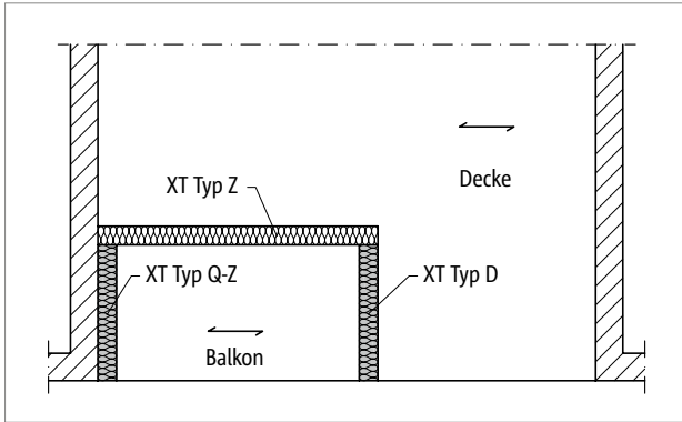
Abb. 309: Schöck Isokorb® XT Typ D, Q-Z: Decke einachsrig gespannt
